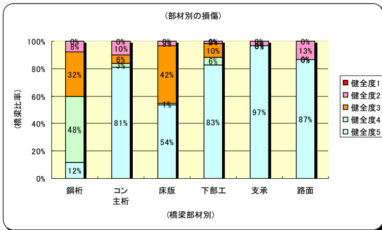
図-部材別の損傷発生状況割合
