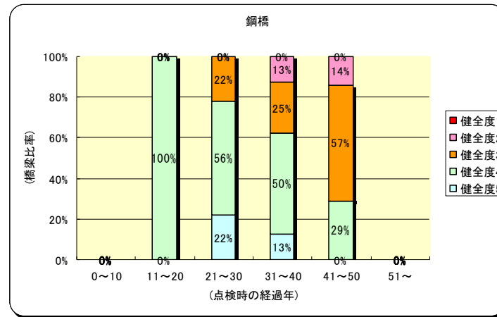
図-鋼橋の経過年別の損傷発生状況割合
